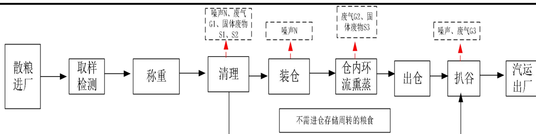
图 2-2 运营期平房仓仓储生产工艺流程及产污节点示意图
