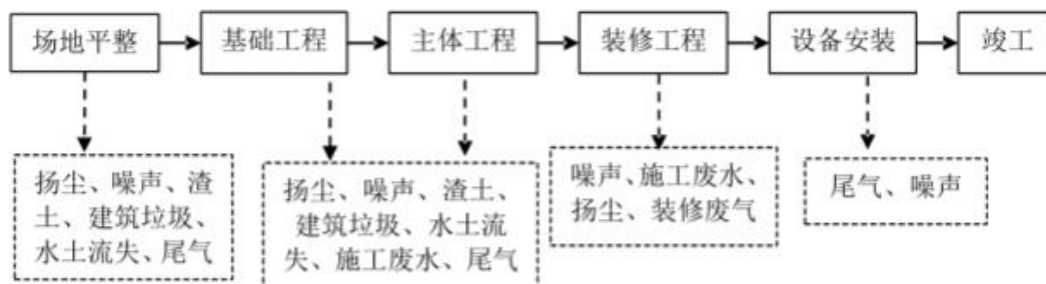
图 2-1 项目施工工艺及产污节点图
