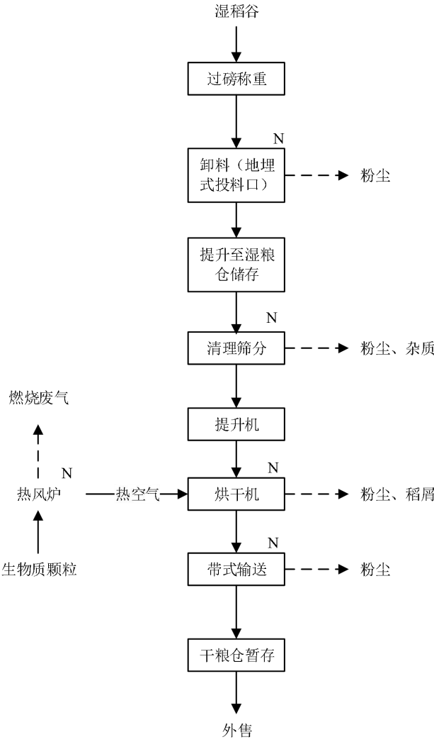
图 2-4 项目运营期湿稻谷烘干生产工艺流程及产污节点示意图
